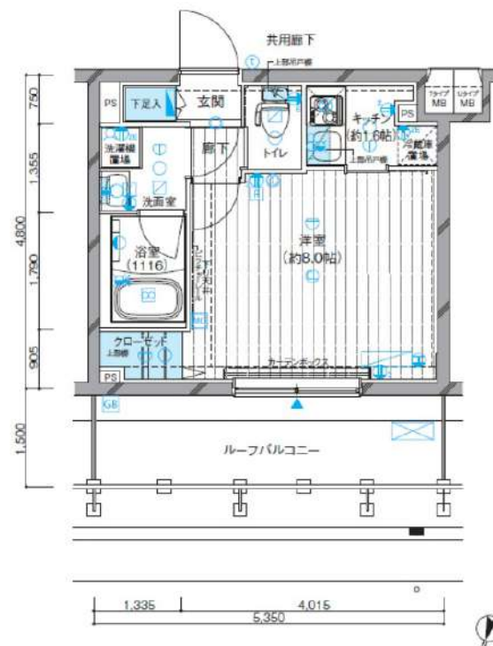
【間取り図】
