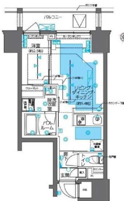
間取り図
