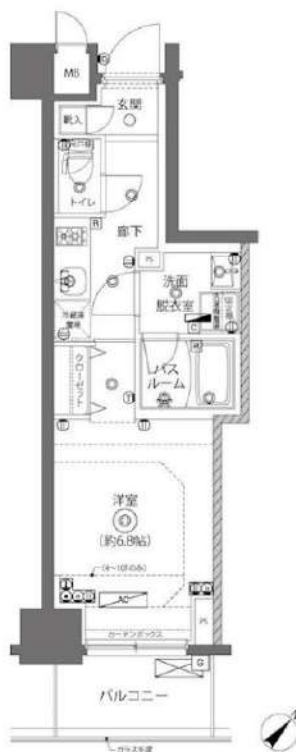
間取り図
