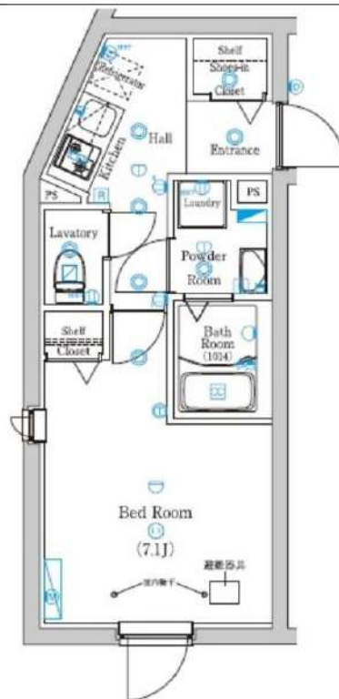
間取り図
