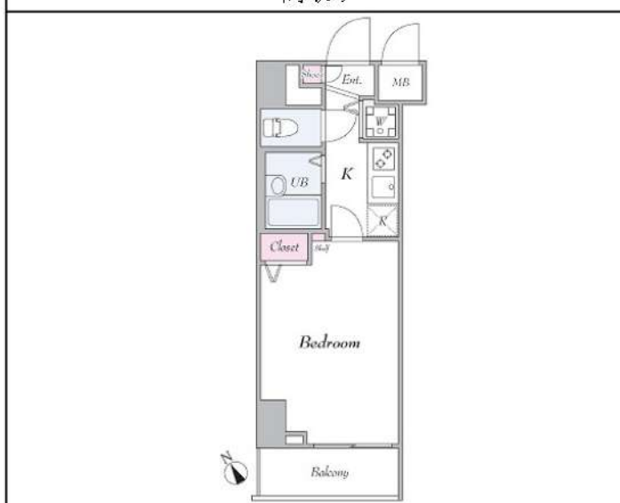
間取り
